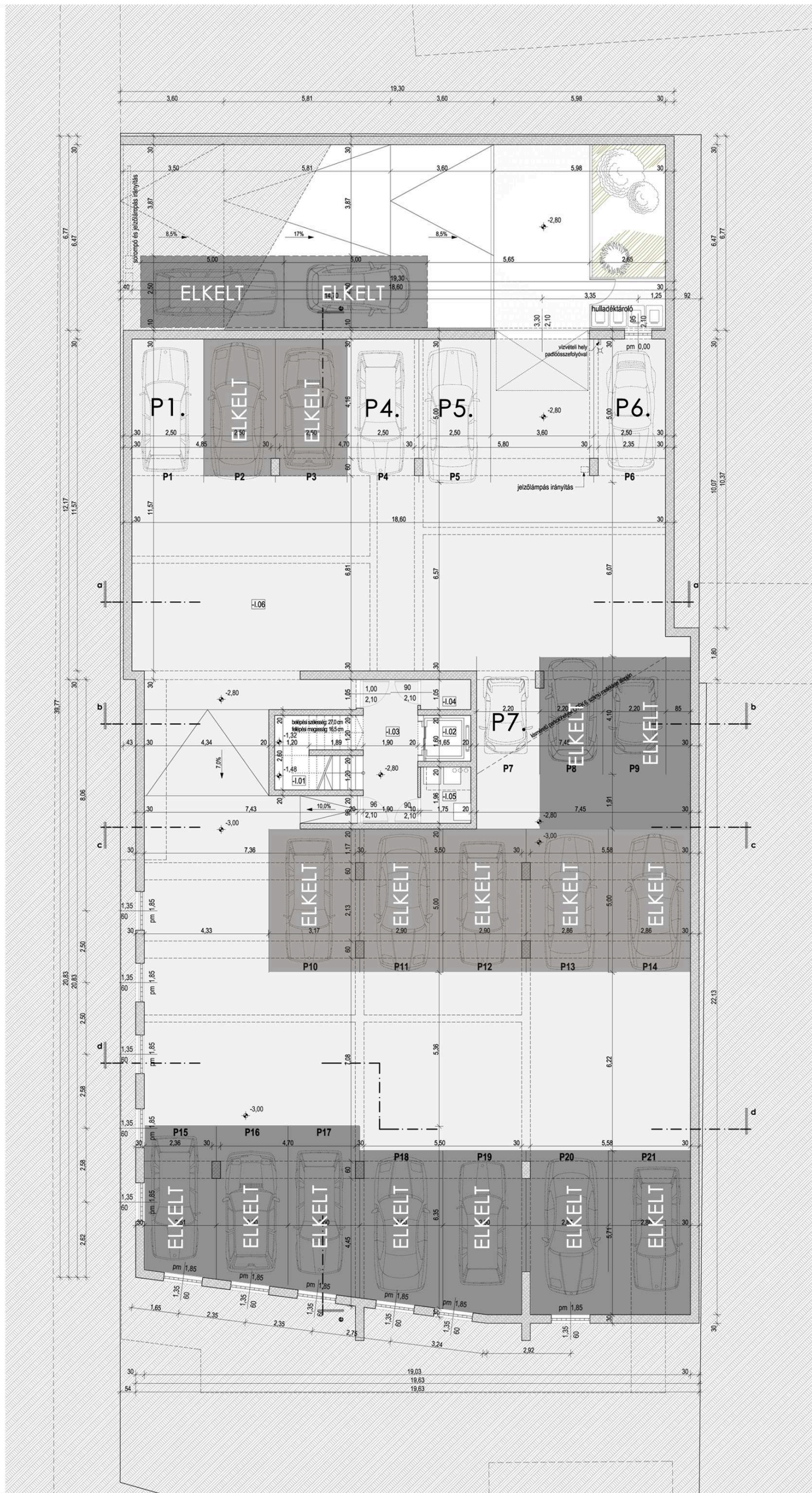
MÉLYGARÁZS ALAPRAJZ_M1:100
